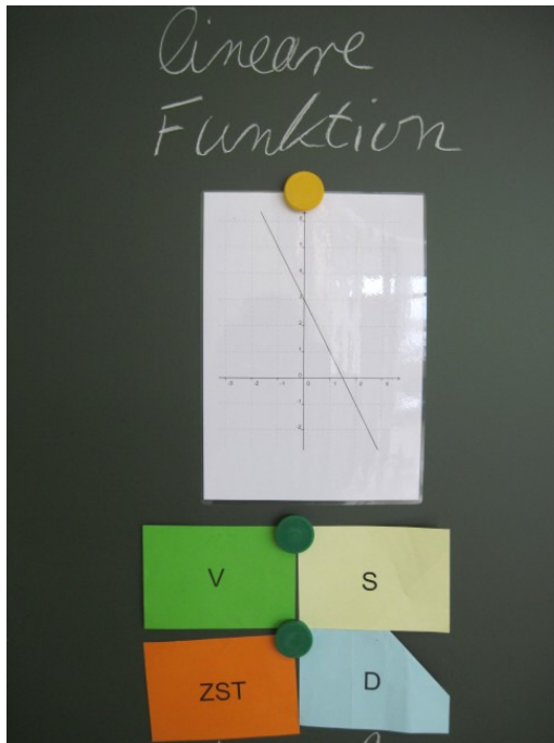
lineare Funktion
