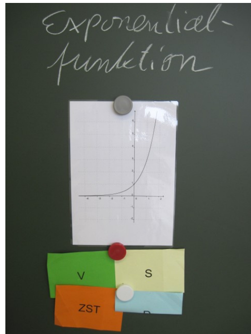
Exponentialfunktion
