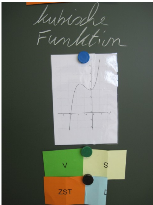
kubische Funktion
