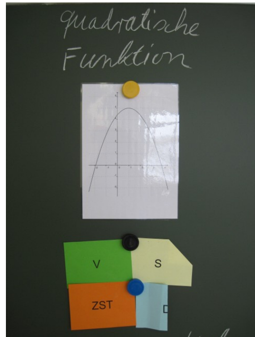
quadratische Funktion
